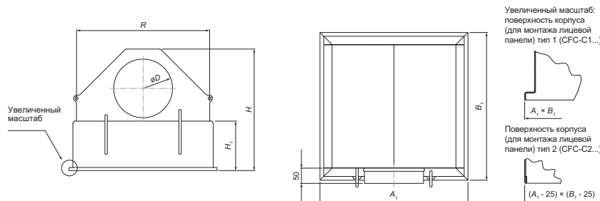
Рис. 2 Корпус CFC-B (Basic)
