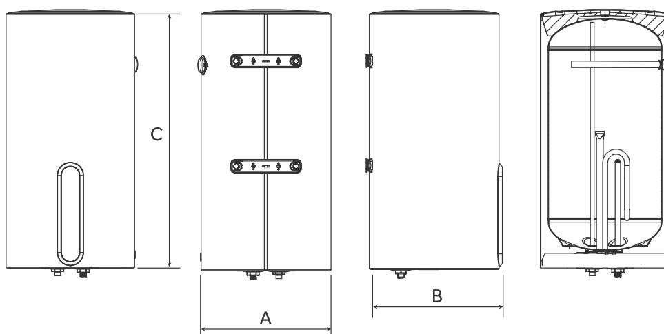
Габаритные размеры (мм)
