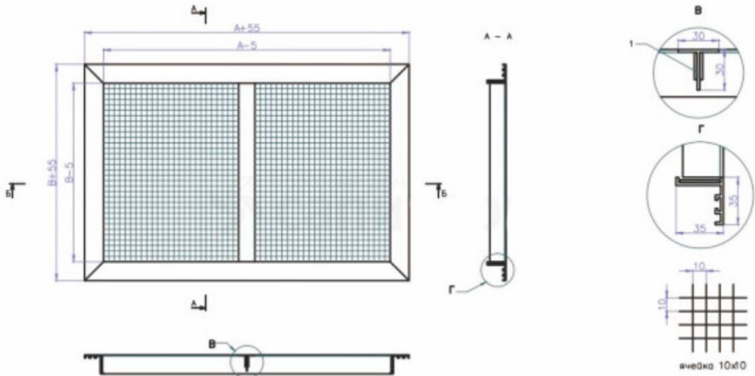
Сетчатая решетка MG АхВ (размер строительного проема)
