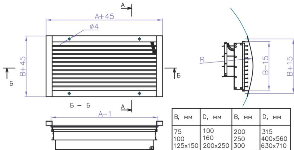
Регулируемая решетка для круглых воздуховодов с регулятором расхода воздуха RGC-R АхВ (размер строительного проема)
