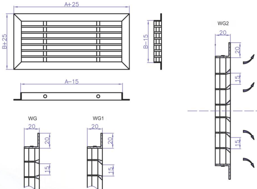
Нерегулируемая приточно-вытяжная решетка WG AxB (размер строительного проема)
