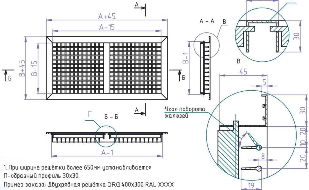
Двухрядная регулируемая решётка DRG АхВ (размер строительного проёма)
