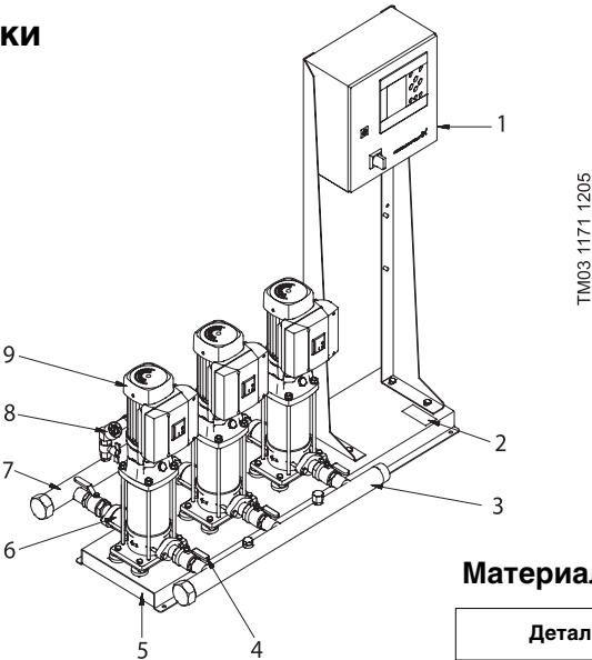
Рис. 1 Конструкция системы
