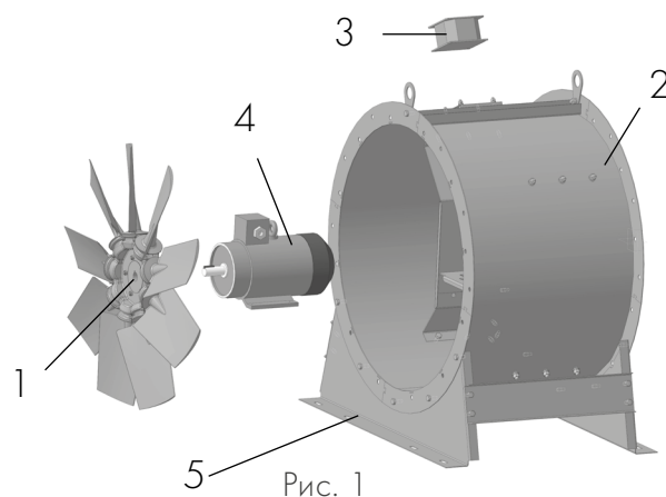
Рис. 1 Устройство осевого вентилятора VO.
