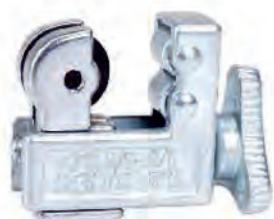
CT-127 Для Ø 1/8"-5/8"
