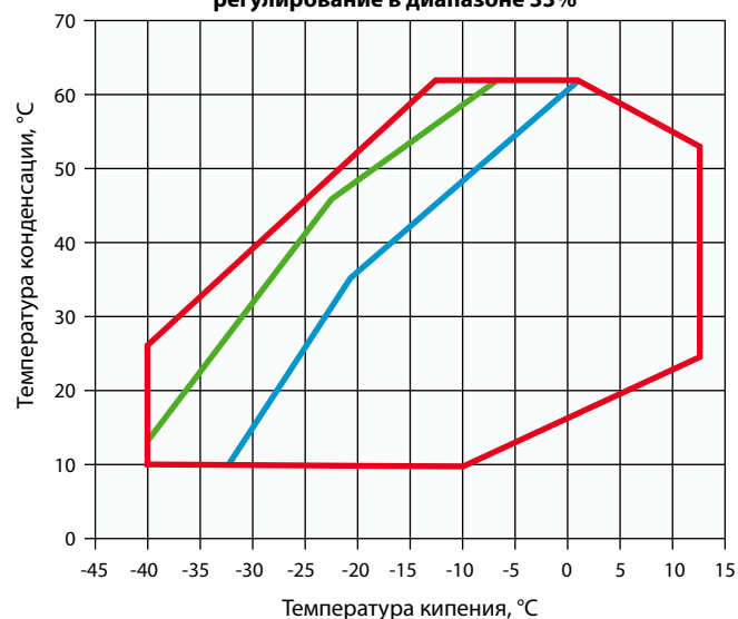
Шестицилиндровый компрессор с большим двигателем – регулирование в диапазоне 33%
