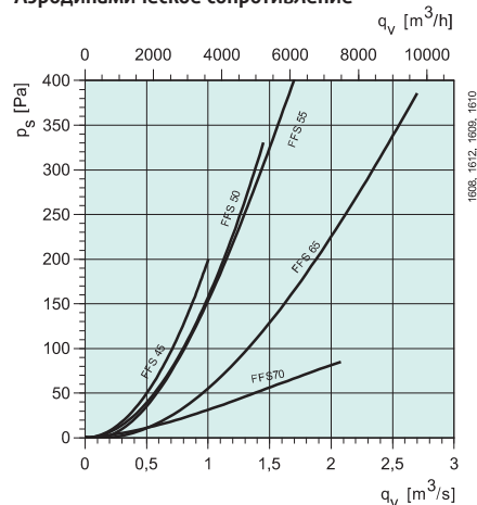
Аэродинамическое сопротивление
