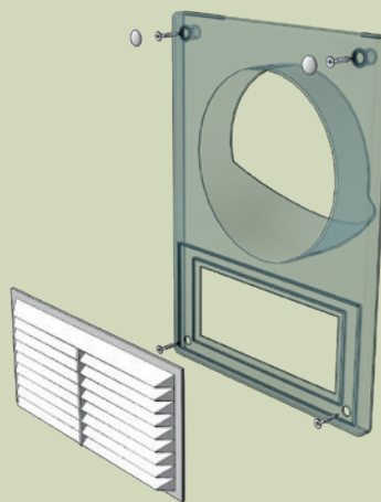
Типовой пример монтажа решётки с помощью шурупов
