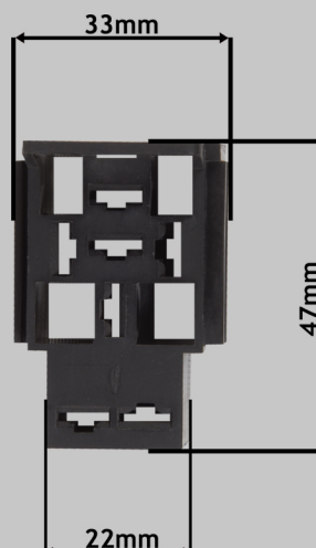
Гнездо реле
